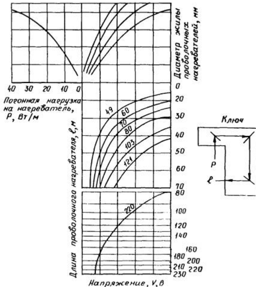
Рис. 3. Номограмма для определения длины проволочных нагревателей
