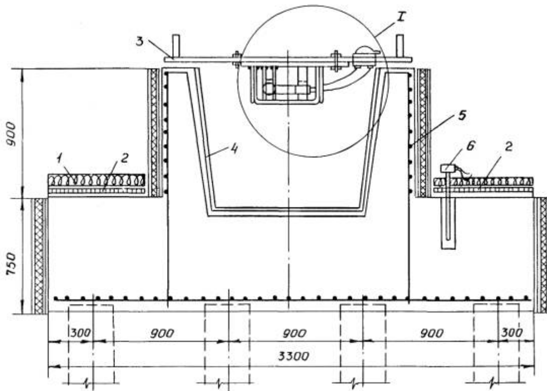
Схема электрообогрева ростверка
