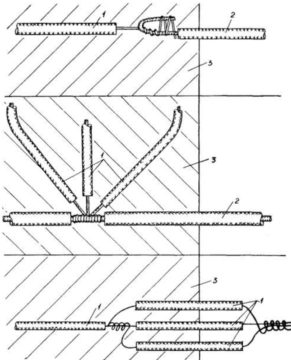
Рис. 4. Выводы нагревательных проводов из бетона:
