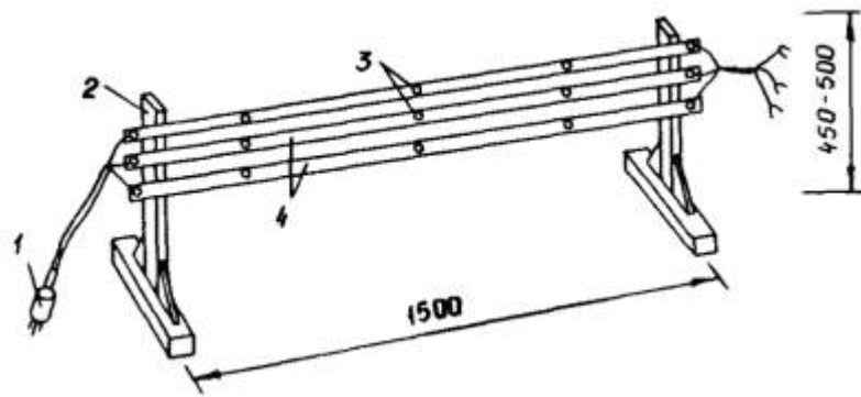
Рис. 2. Инвентарная секция шинопроводов (крайняя секция):
