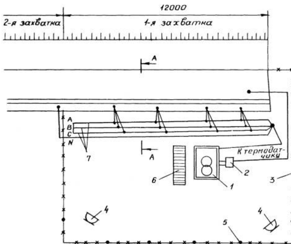
Схема электрообогрева подпорной стенки
