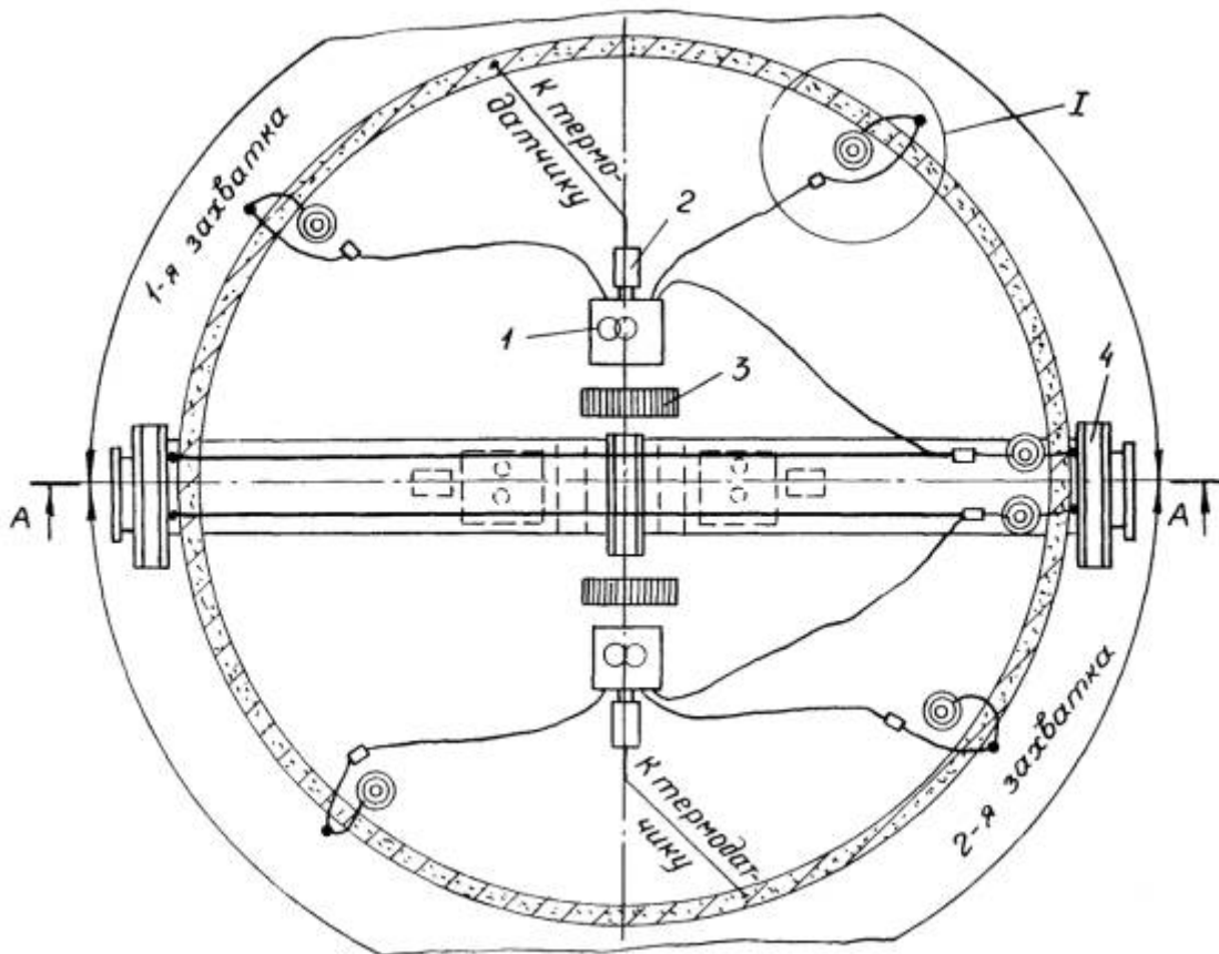
Схема электрообогрева гиперболической градирни
