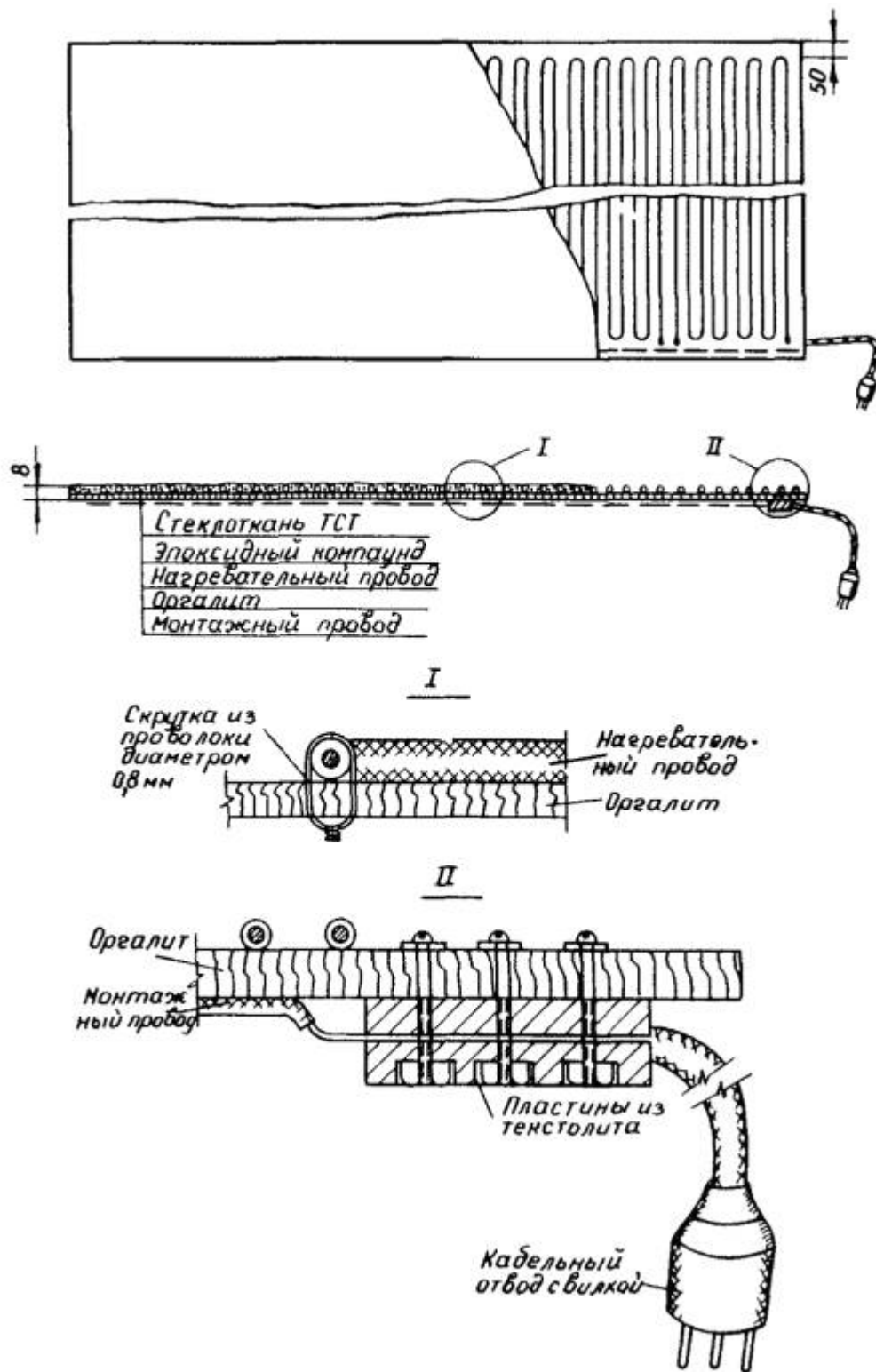
Рис. 1. Греющий плоский элемент (ГЭП)
