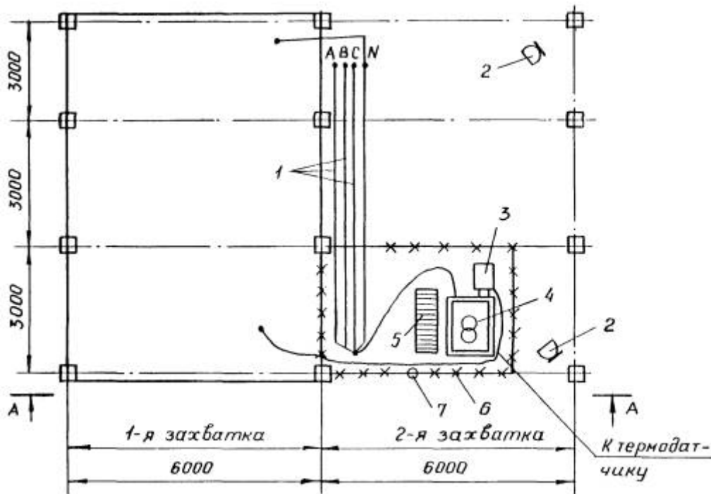
Схема электрообогрева плит перекрытия
